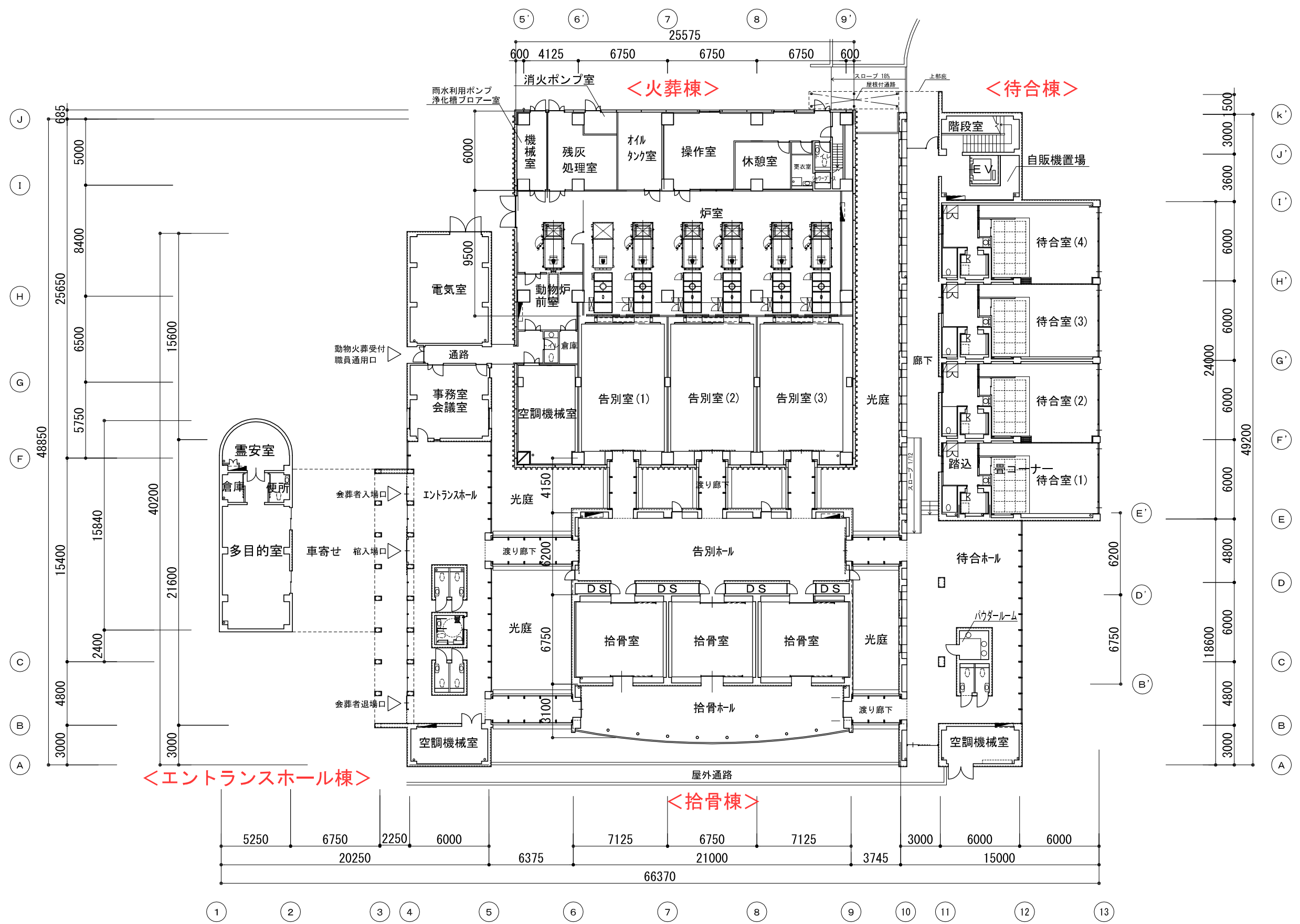
1 階 平 面 図
