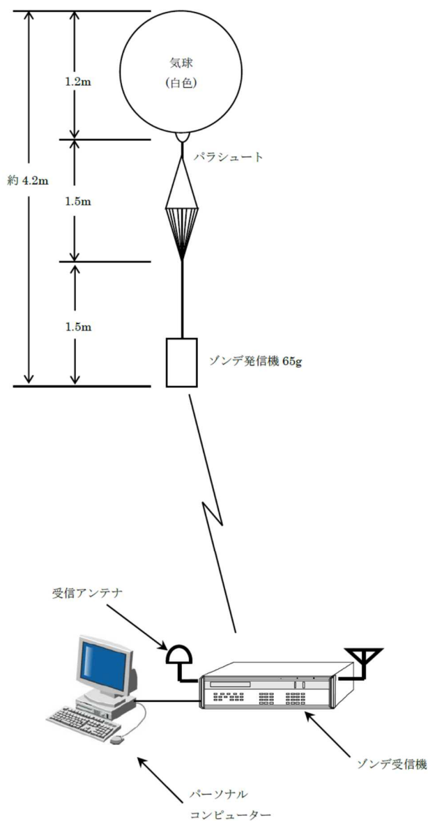
図 2 GPS ゾンデによる上層気象観測概略図
