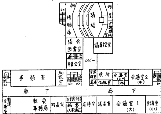
2階 平面図
