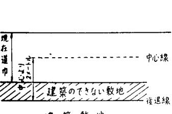
図2 平面図
