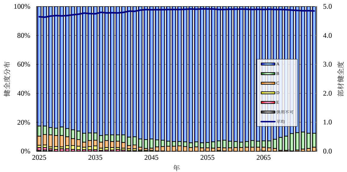
健全度分布の推移（主部材のみ）
