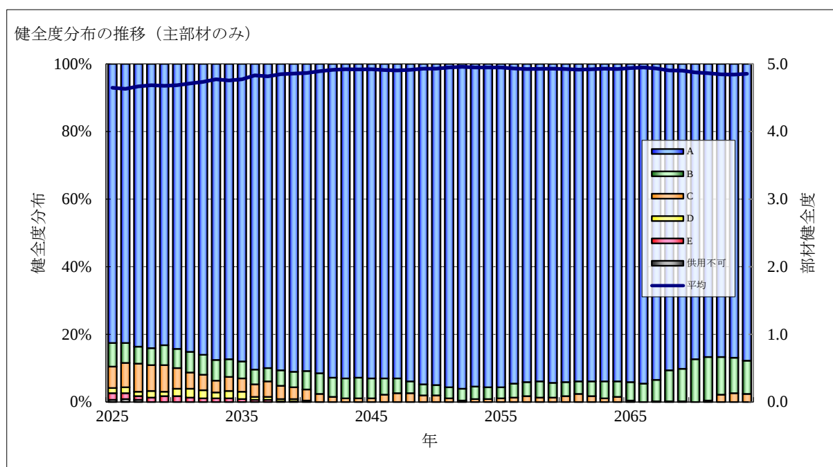
図3-22 主部材別健全度分布の推移
