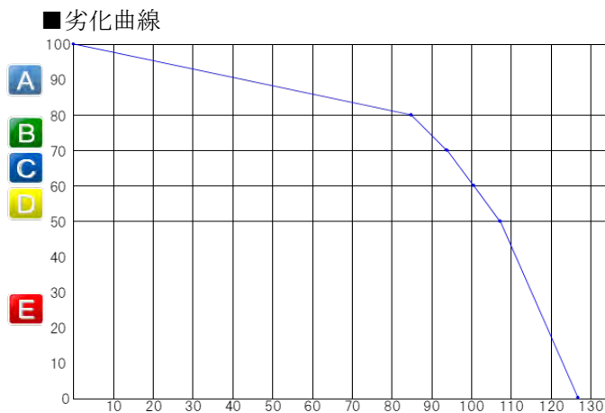
図2-10 劣化曲線(7)
