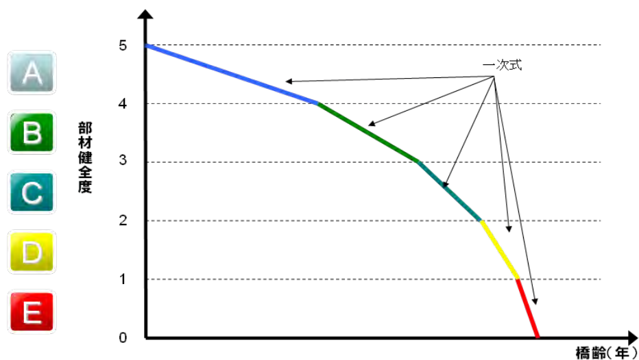
図2-2 劣化過程のイメージ
