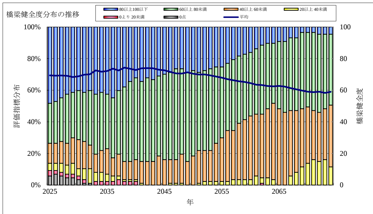
図3-20 橋梁別健全度分布の推移
