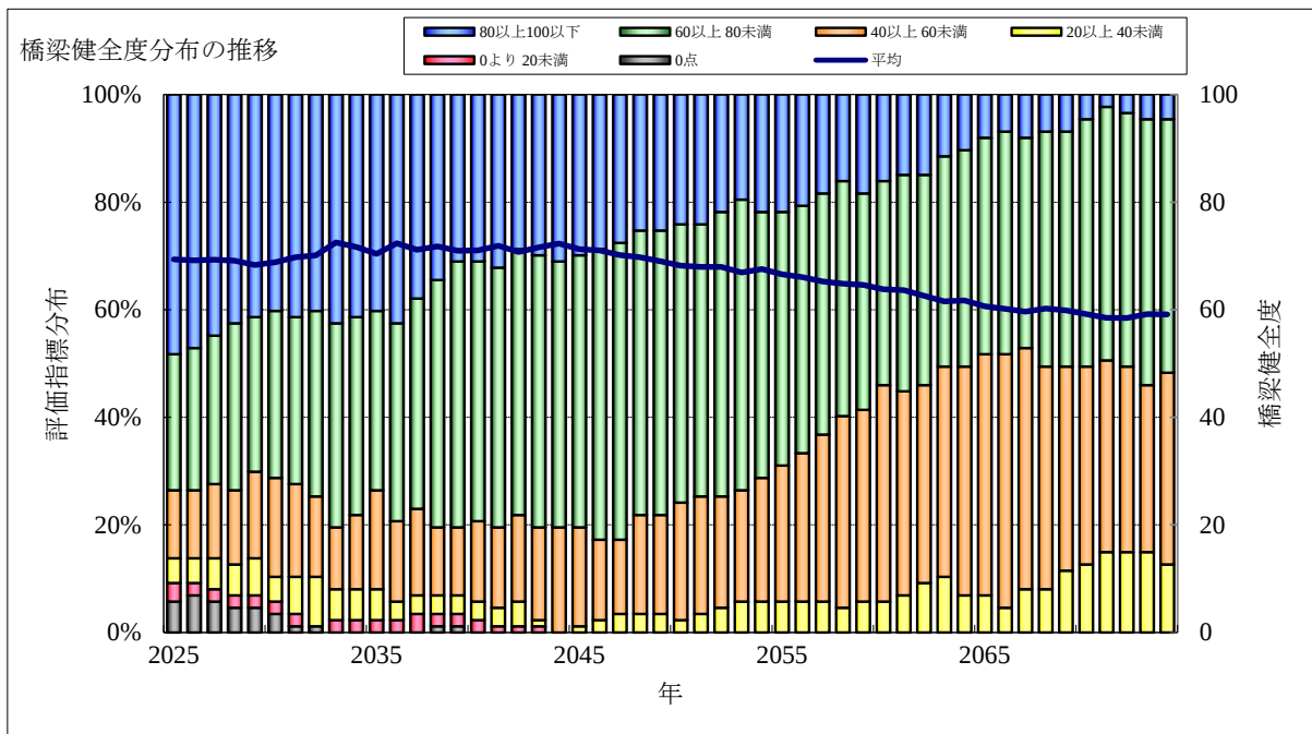
図3-24 橋梁別健全度分布の推移
