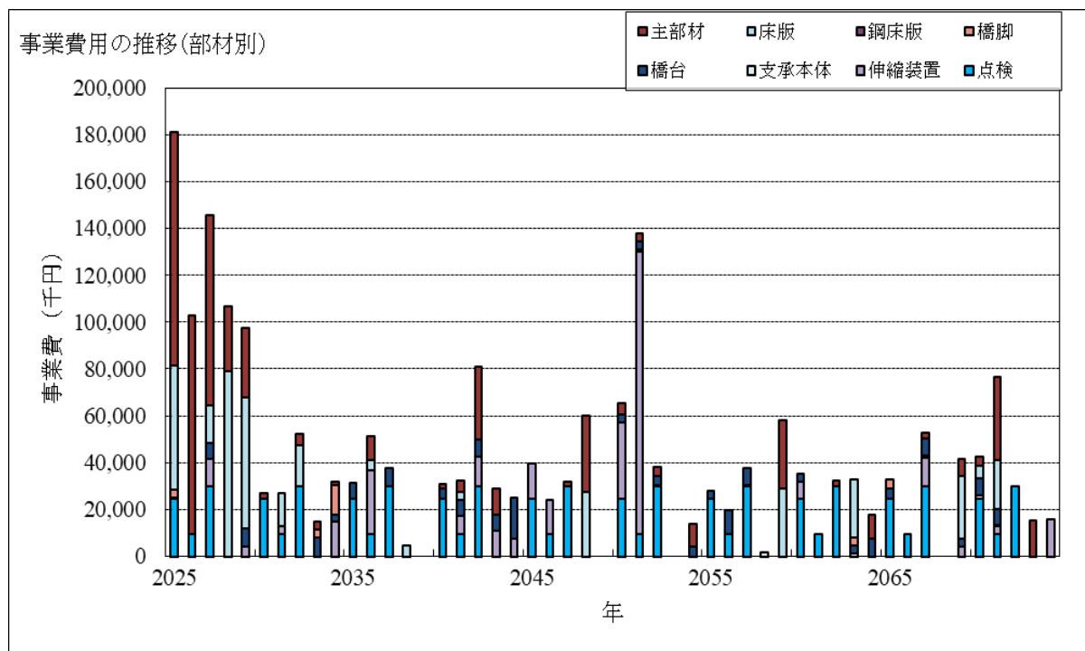
図3-5 部材別事業費の推移
