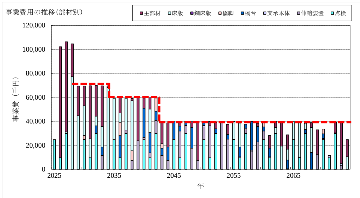
図3-23 部材別事業費の推移
