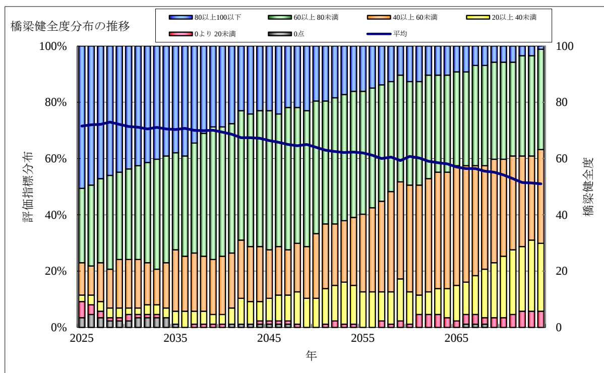
図3-10 橋梁健全度分布の推移
