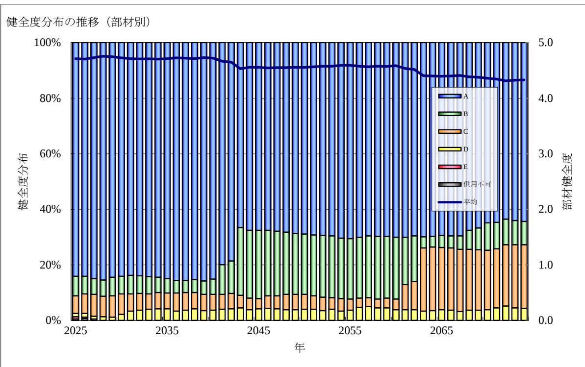
図3-11 部材別健全度分布の推移
