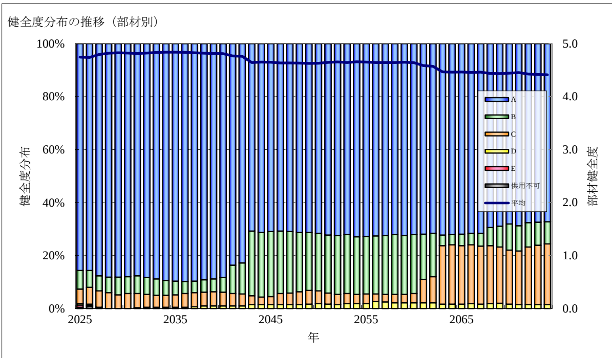
図3-7 部材健全度分布の推移
