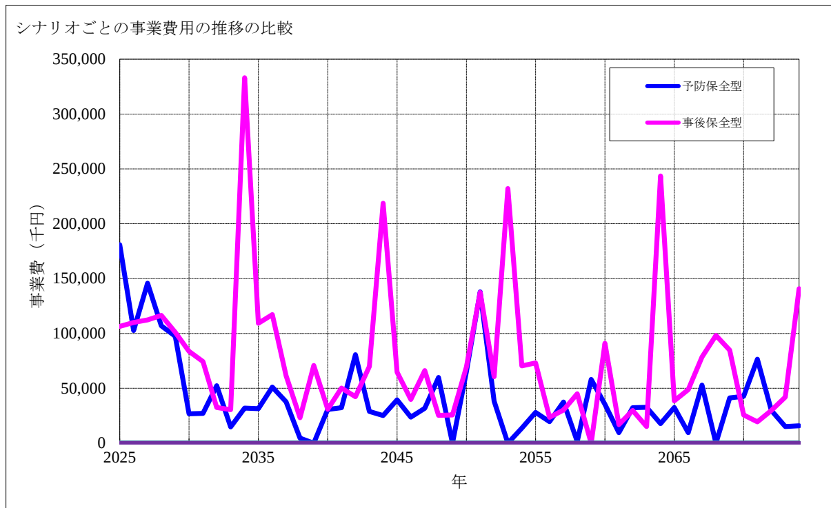
図3-3 事業費の推移の比較
