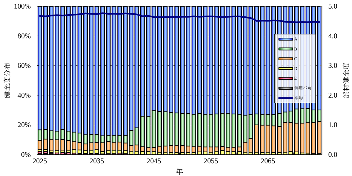
健全度分布の推移（部材別）
