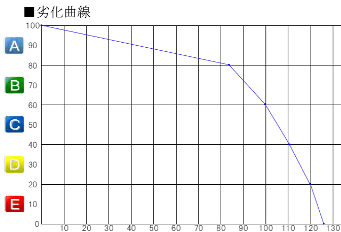
図2-11 劣化曲線(8)
