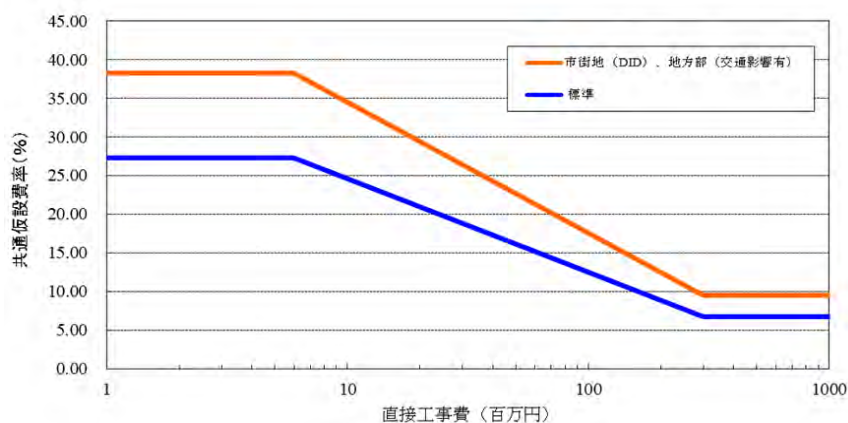
図2-14 直接工事費と共通仮設費率の関係
