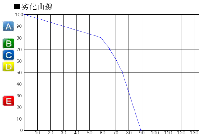
図2-7 劣化曲線(4)
