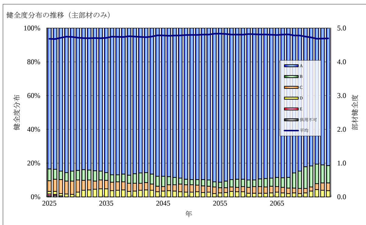
図3-12 主部材健全度分布の推移
