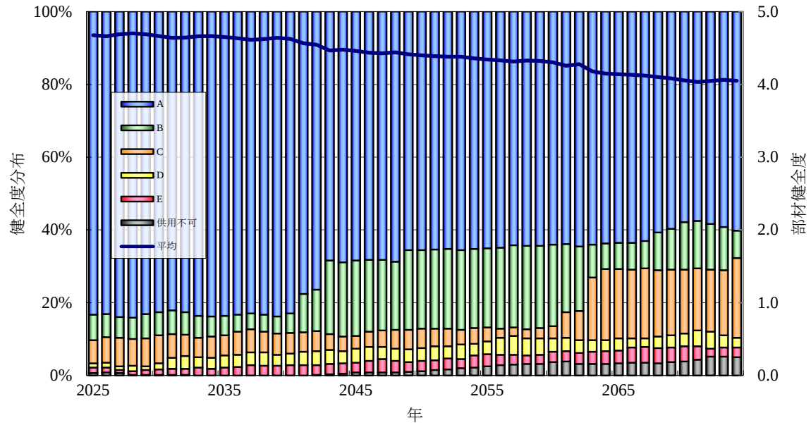
健全度分布の推移（部材別）
