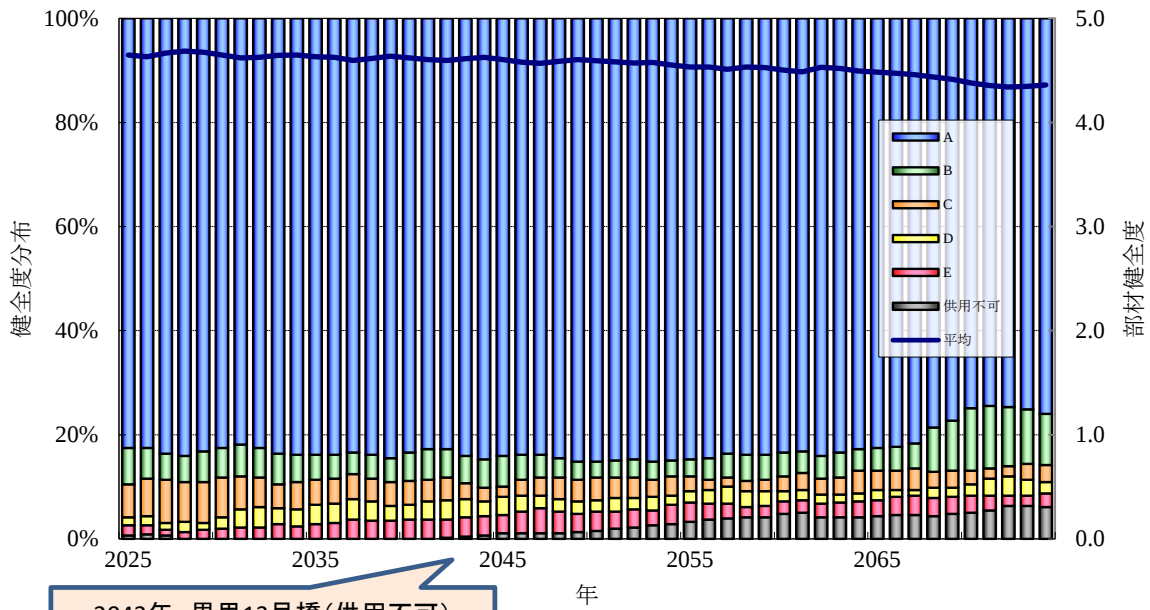
健全度分布の推移（主部材のみ）
