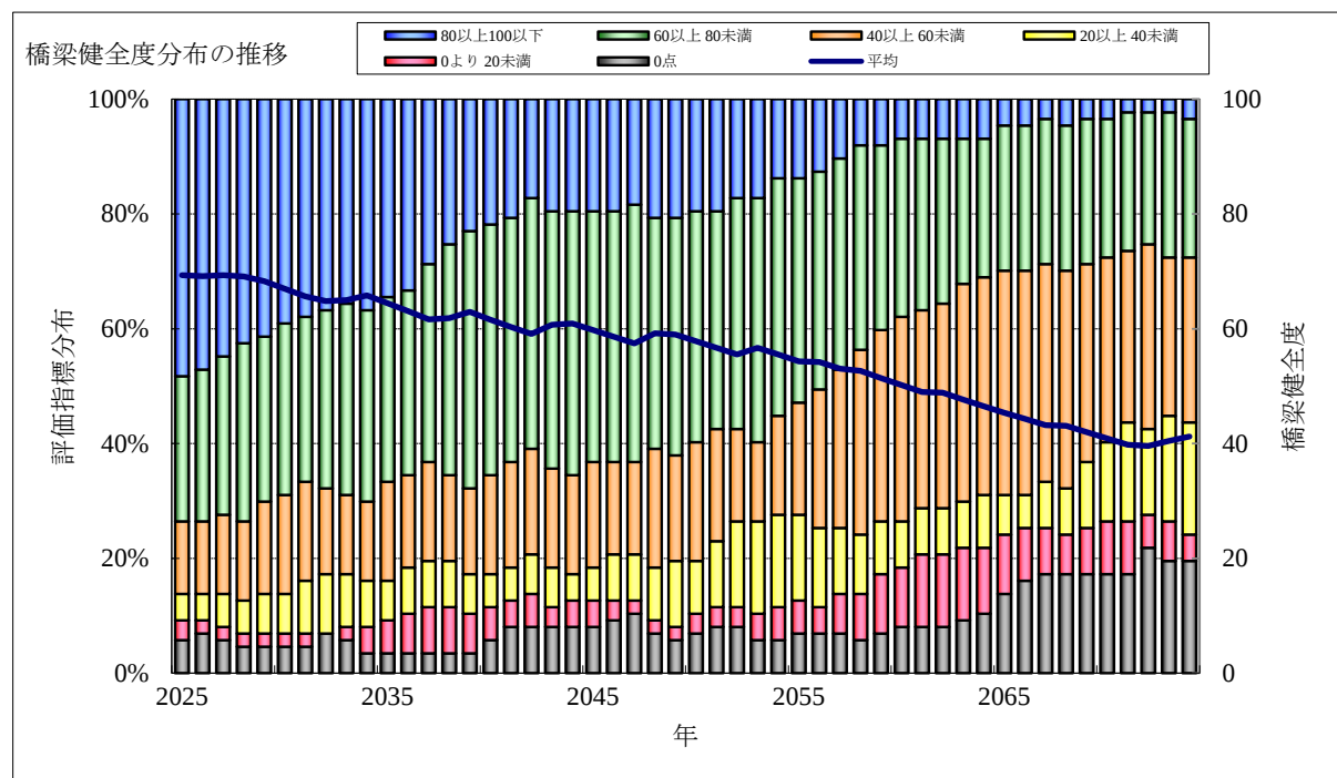
図3-16 橋梁別健全度分布の推移
