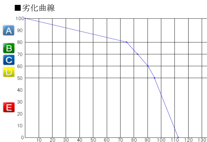
図2-9 劣化曲線(6)
