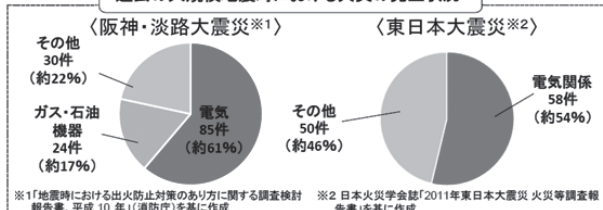
過去の大規模地震時における火災の発生状況
